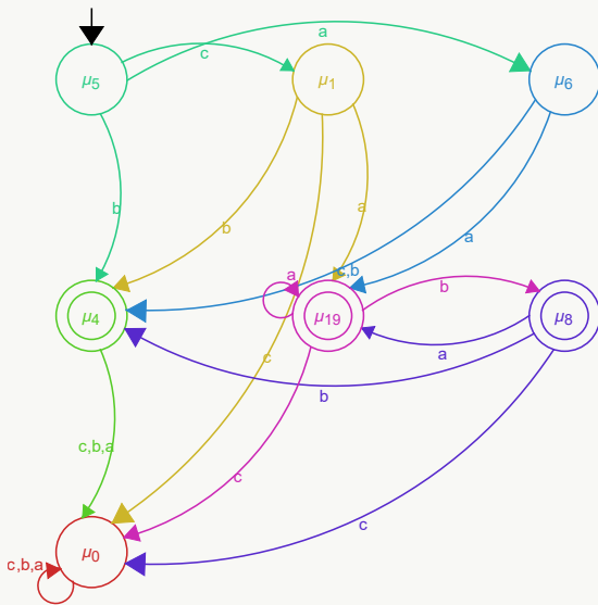
Diagrama de transición reducido del nuevo autómata:
