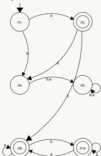
Diagrama de transición reducido del nuevo autómata:
