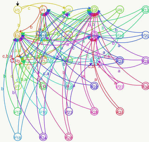
Diagrama de transición reducido del nuevo autómata:
